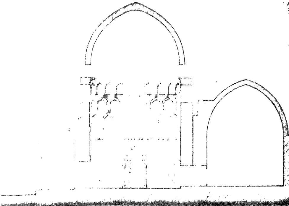
لوحة (١١٩) التفاصيل الداخلة لقبة الصالح نجم الدين
